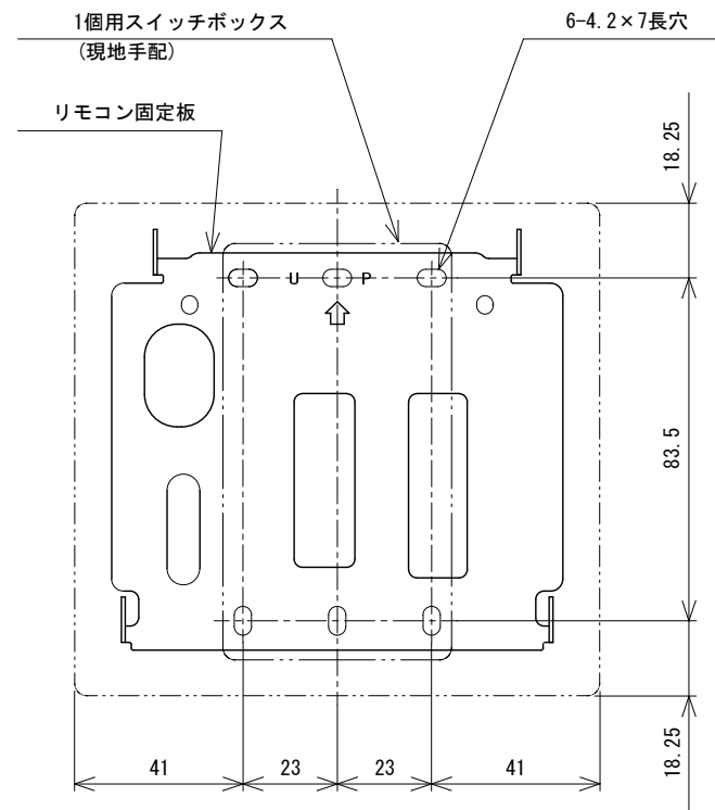
取付金具
