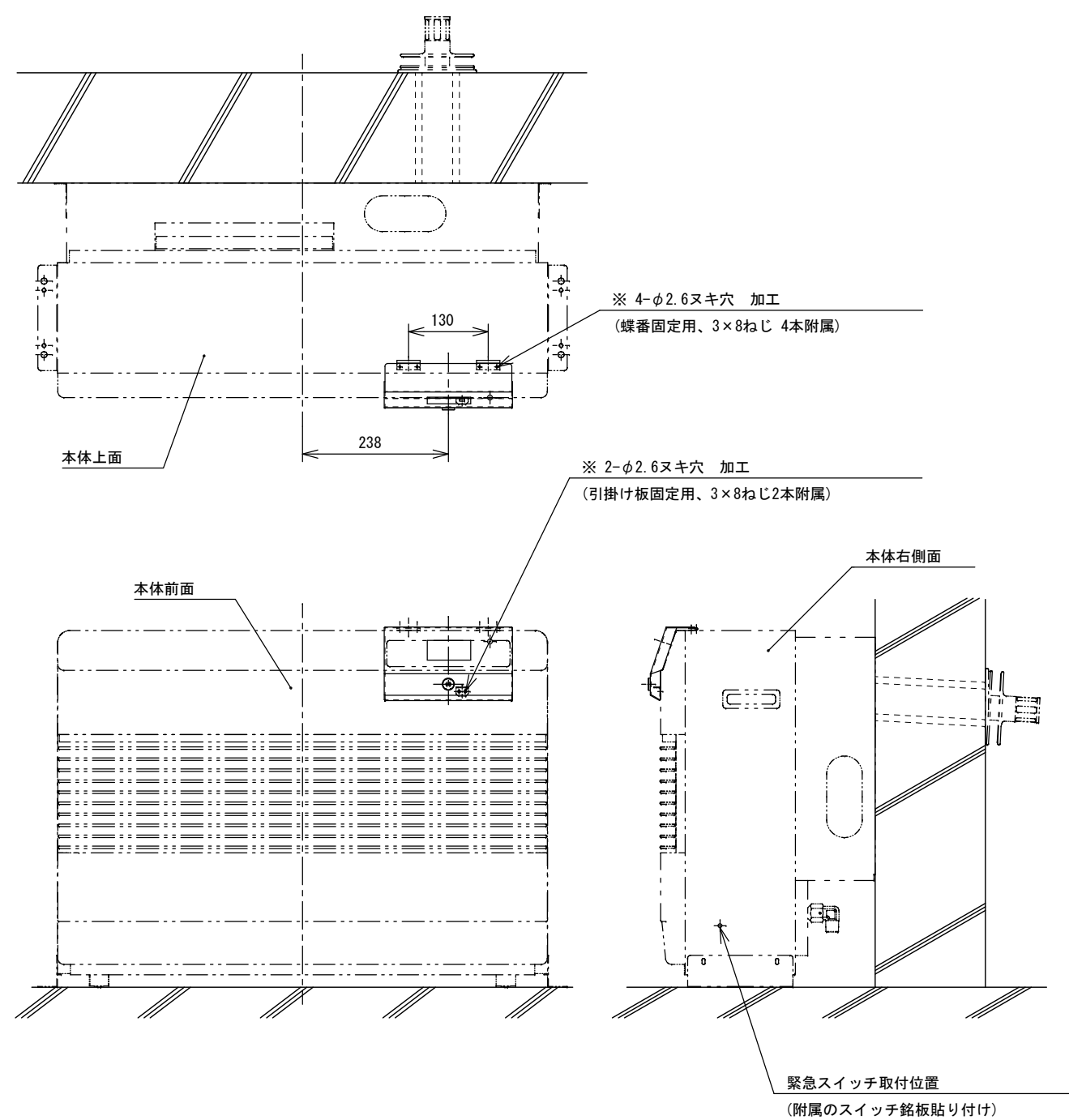
カギ付パネル本体 引掛け板 取付穴位置寸法
