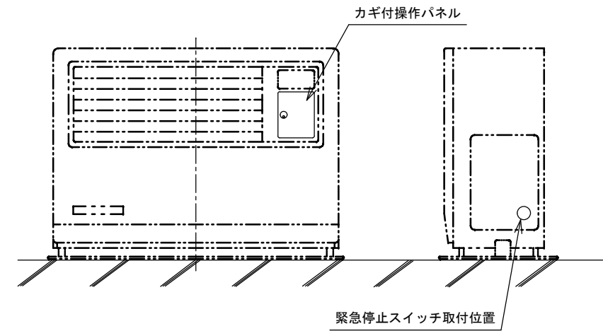
カギ付操作パネル取付位置
