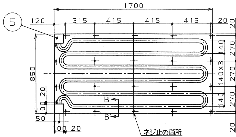
FHP-12WSB 1:20
