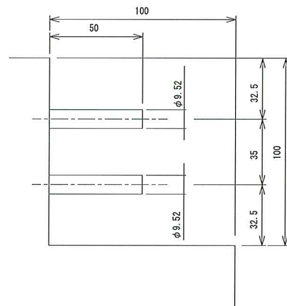
B部詳細図 1/2
