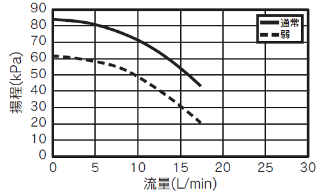
機外揚程表
