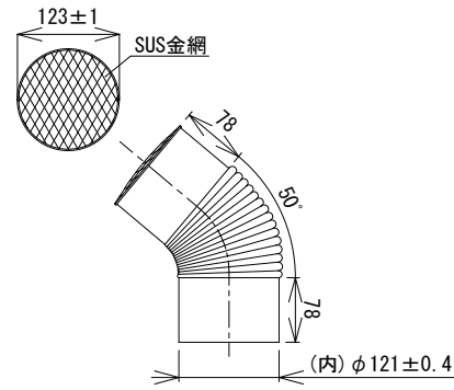
(参考) 別売品網付エルボトップ詳細
