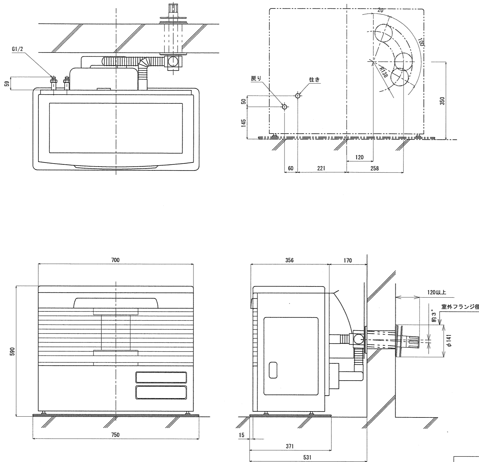
標準給排気筒穴位置(正面図)
